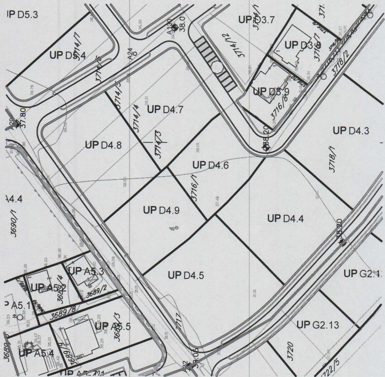
Planski trafo reon 10, planirana trafostanica TS 10/0.4kV/kV "7", 1x1000kVA
