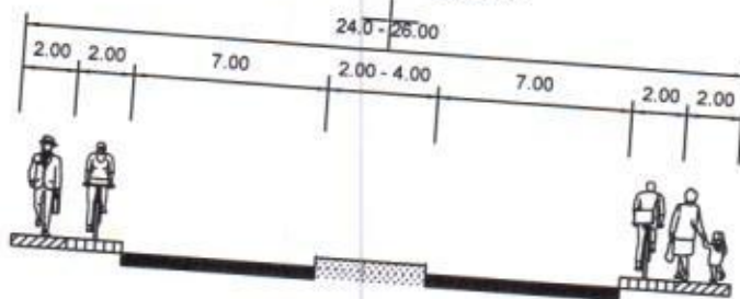
presjek 8-8
