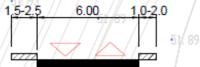
presjek 21-21
